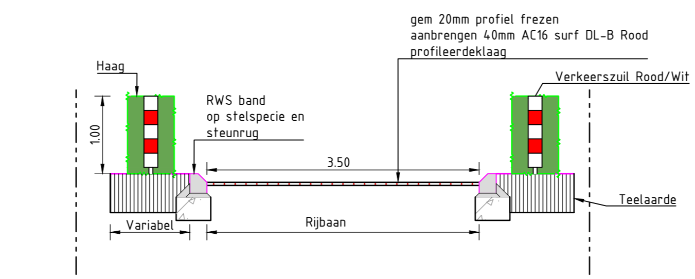
Principeprofiel B-B
