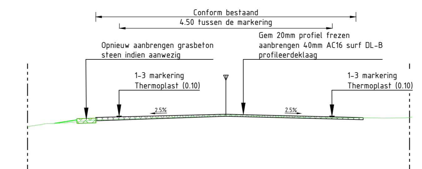
Principeprofiel
