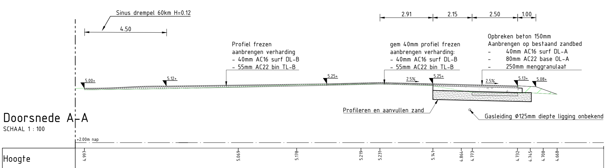
Doorsnede A-A
